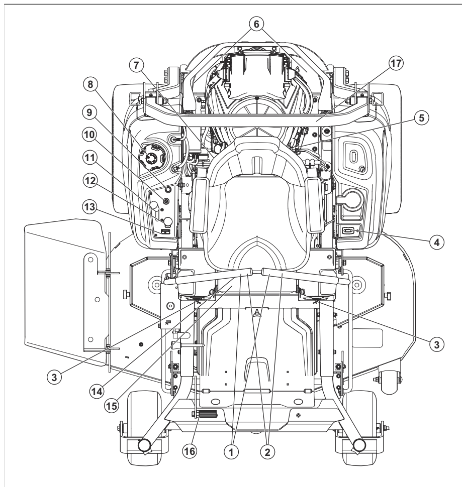
1. Ovládací páky
